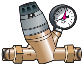
Réducteur de pression équipé d'un manomètre (coût matériel ≈ 30€)
