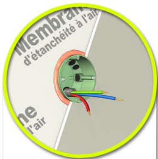
Pose d'un boîtier électrique plein
