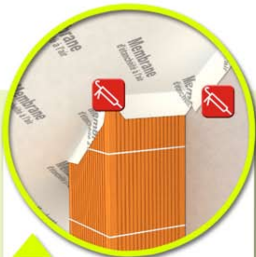
Raccordement sur boisseaux isolés
