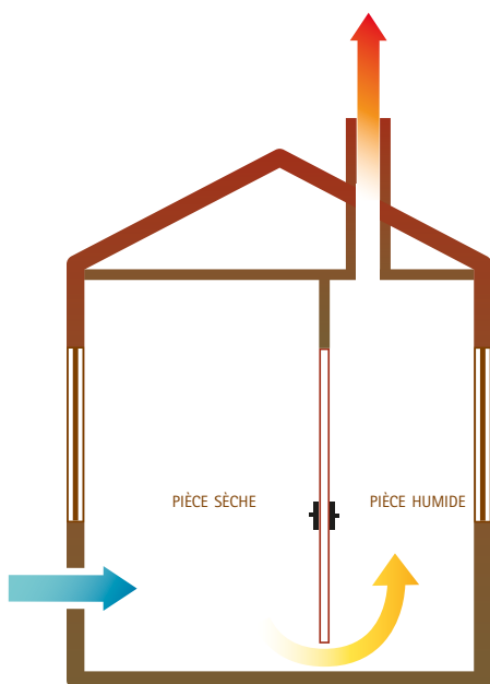
> PRINCIPE DE FONCTIONNEMENT DE LA VENTILATION NATURELLE.
