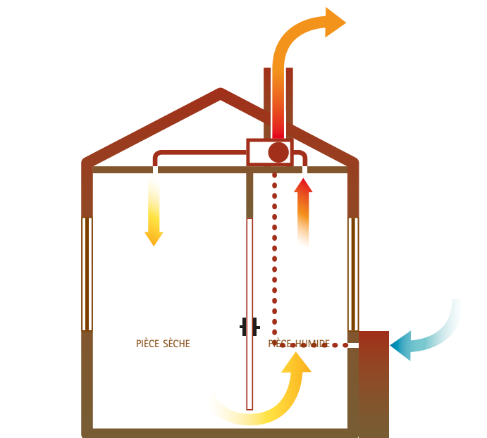
> FONCTIONNEMENT D'UN CAISSON VMC DOUBLE FLUX COUPLÉ À UNE CHAUDIÈRE GAZ
