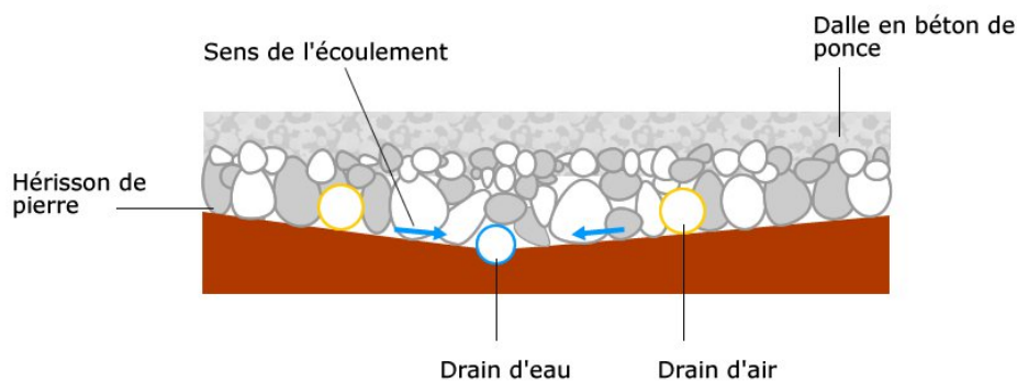
Montage d'une dalle de rez-de-chaussée en milieu humide Coupe transversale
