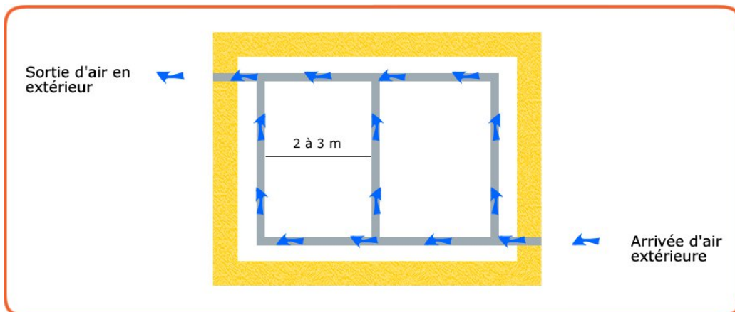
Positionnement du drain d'air Vue de dessus
