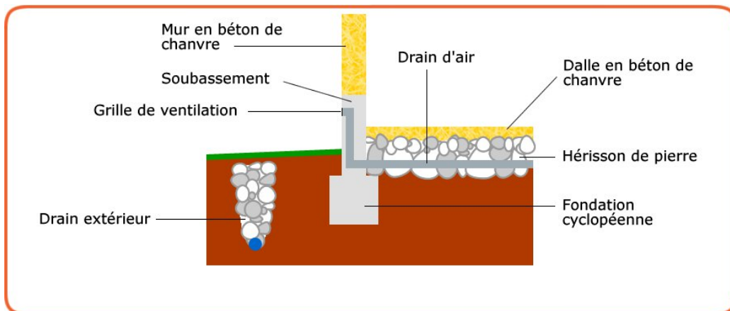
Protection du hérisson des entrées humides extérieures Coupe longitudinale
