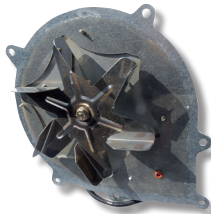
Extracteur de fumée démonté
