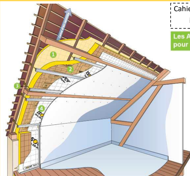
La Source : schéma Isover « isolation pour les combles aménagés »
