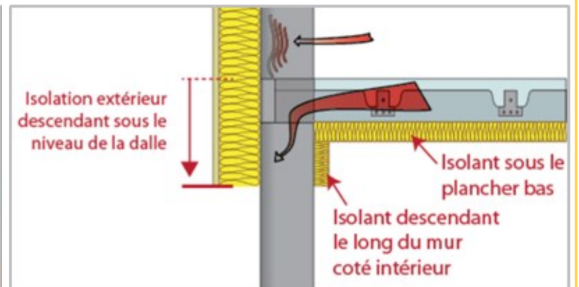
Isolation descendant sous le niveau de la dalle (limite les ponts thermiques) surtout si retour côté intérieur
