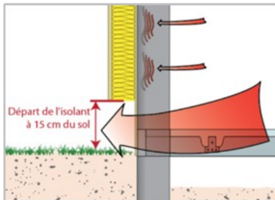
Démarrage de l'isolation à 15 cm du sol = pont thermique
