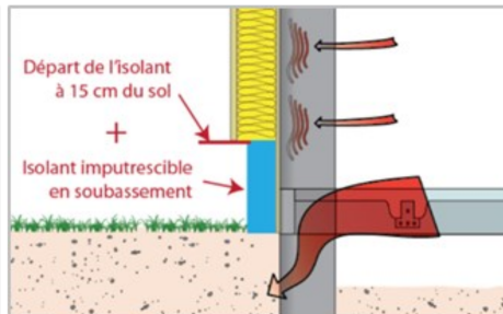
Continuité de l'isolation jusqu'au sol ou semi-enterré = pas de pont thermique
