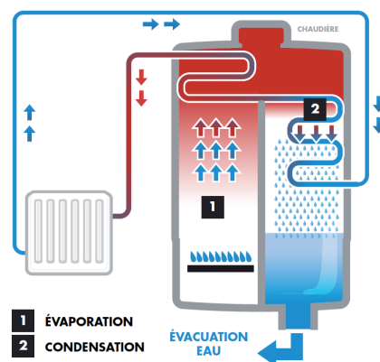
Fonctionnement de la chaudière à condensation
